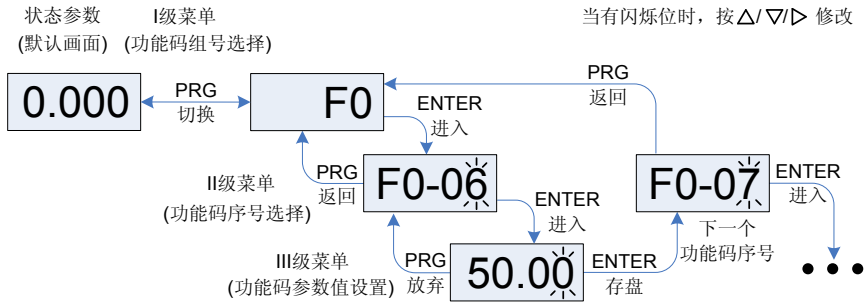
图 4-4 三级菜单操作流程图
