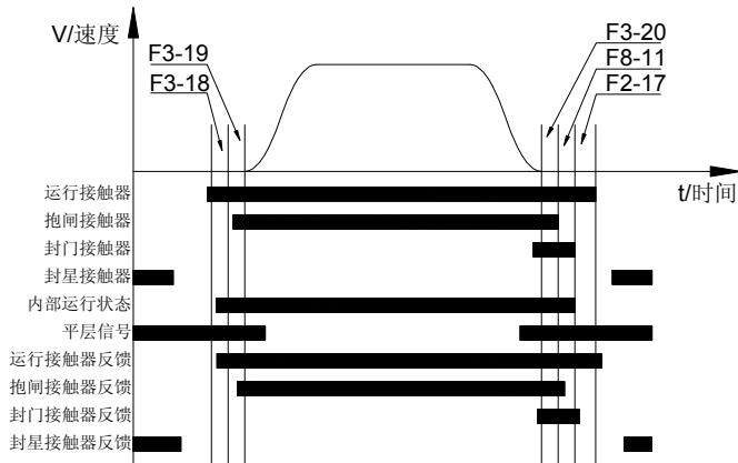
图 7-3 运行时序图
