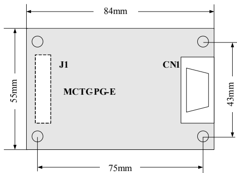
图3-9 MCTC-PG-E尺寸图
