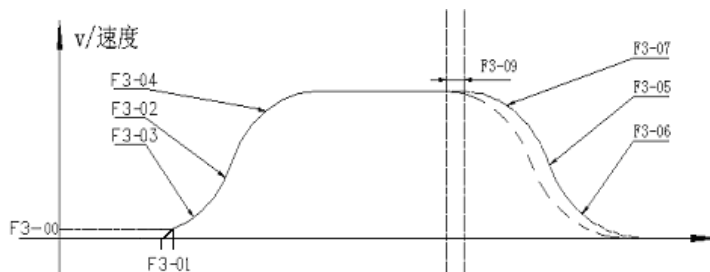
图6-3 速度曲线图
