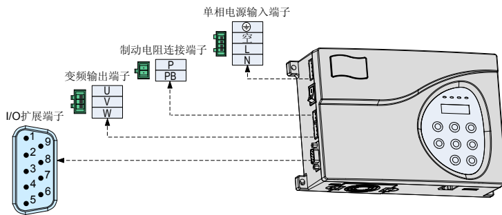
图 3-1 驱动回路端子分布图
