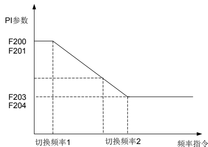
图 6-1 PI 参数示意图
