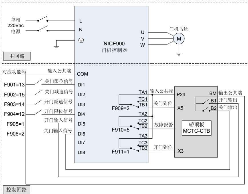
图 4-10 速度控制系统典型应用接线图
