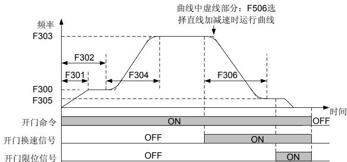
图 6-3 速度控制开门曲线示意图
