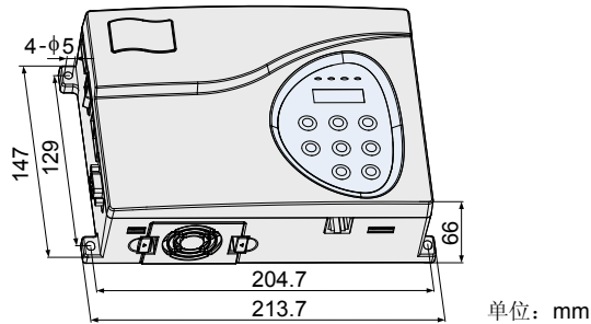
图 2-3 产品外型尺寸图
