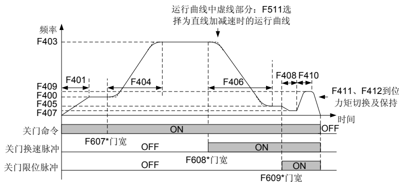
图 6-6 异步门刀距离控制关门曲线示意图
