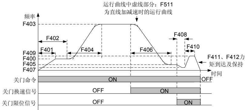
图 6-5 速度控制关门曲线示意图
