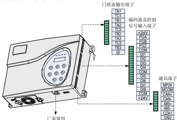
图 3-3 控制回路端子分布图
