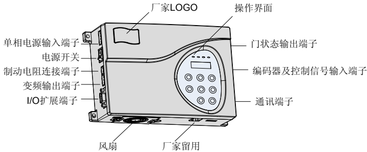
图 2-1 产品外观图
