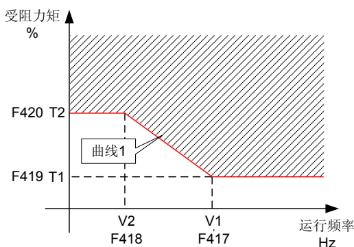
图 6-7 关门受阻判断示意图
