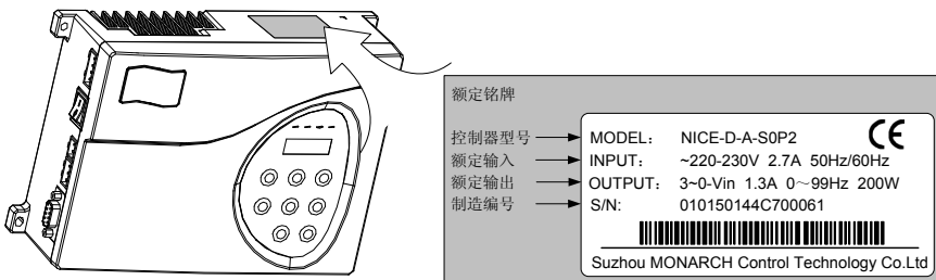
图 2-2 铭牌举例
