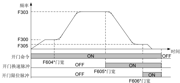
图 4-15 距离控制开门曲线示意图
